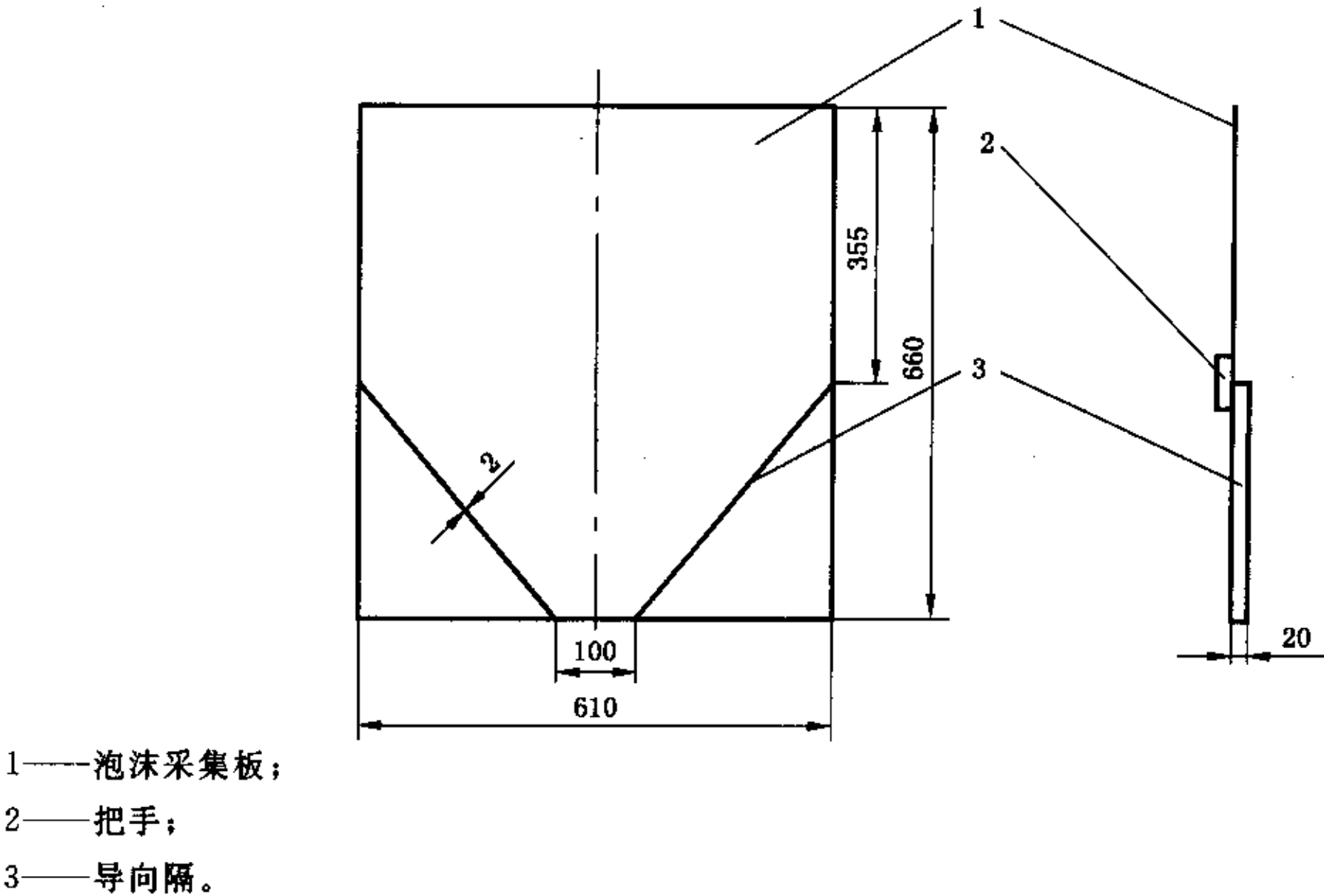
图 1 泡沫采集器
